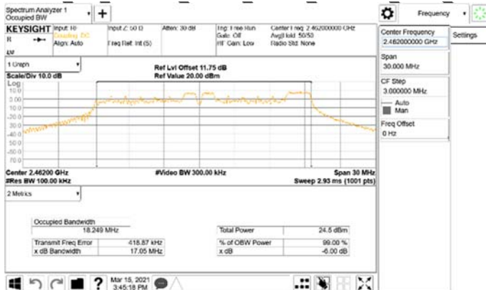
6dB_BW_802.11ax_20MHz_Chain0_2462MHz_RU52_40
