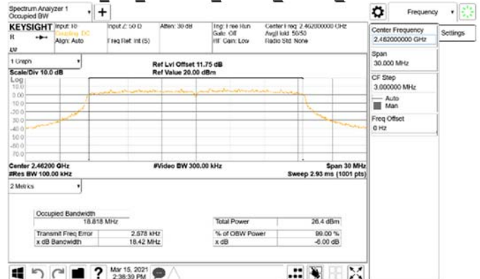
6dB BW_802.11ax_20MHz_Chain0_2462MHz
