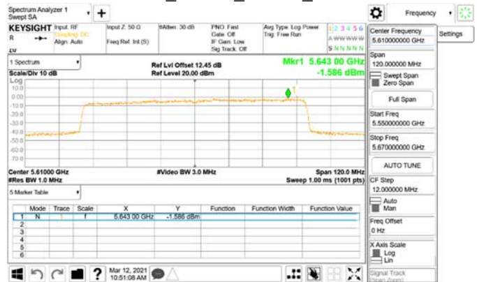
802.11ax_80MHz_Chain0_5610MHz_RU484_66
