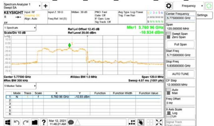
802.11ax_80MHz_Chain1_5775MHz_RU484_66
