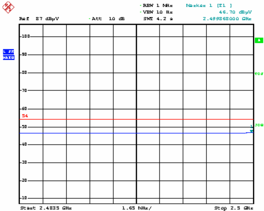
802.11b high channel Hor AV
