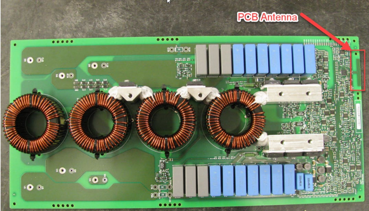
PCBA Top
