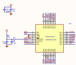
MCU module-1
