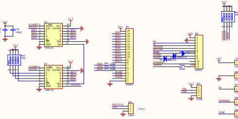
Interface module
