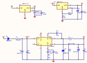
Power Module
