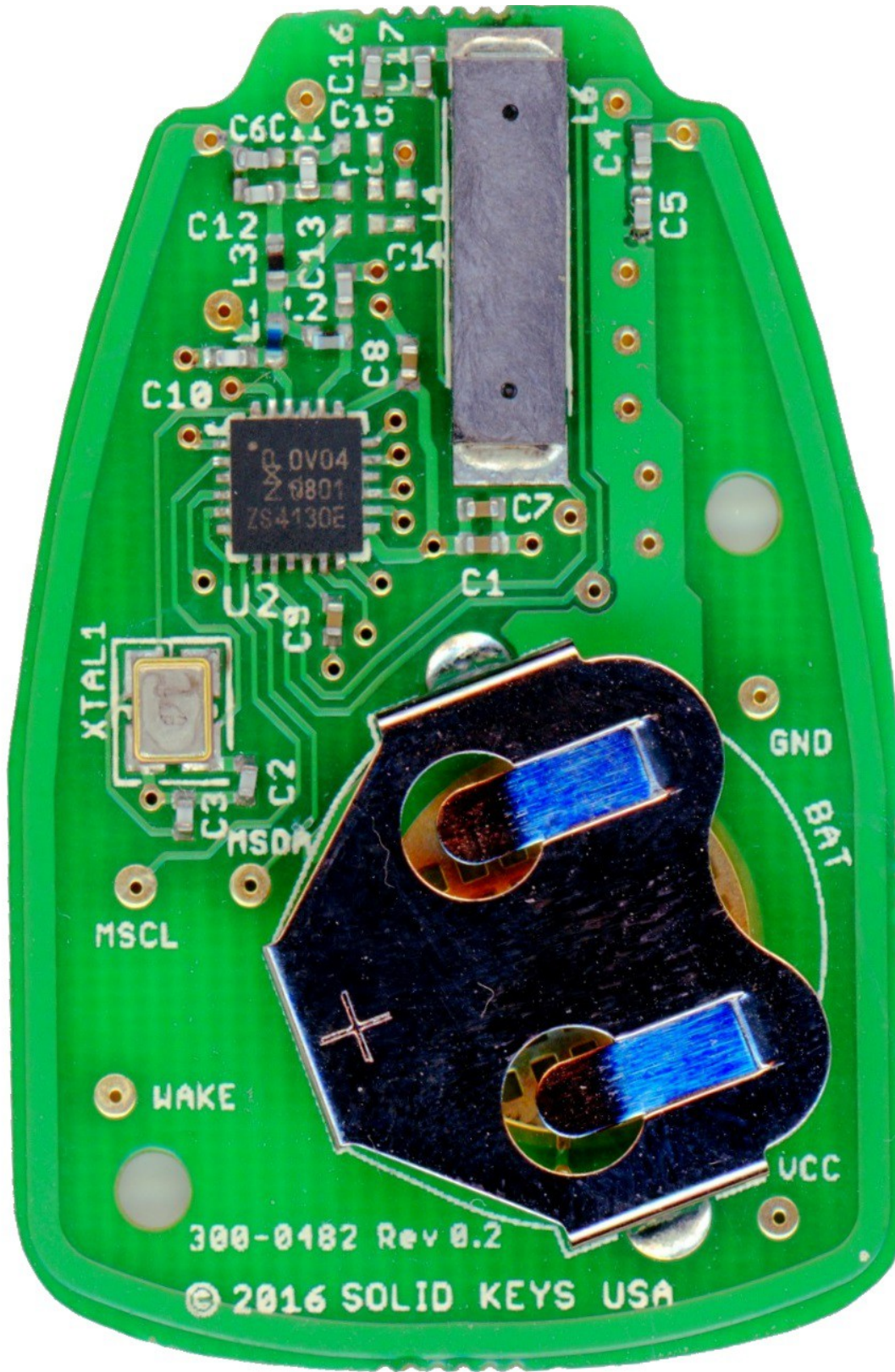
300-0482 PCB Top
