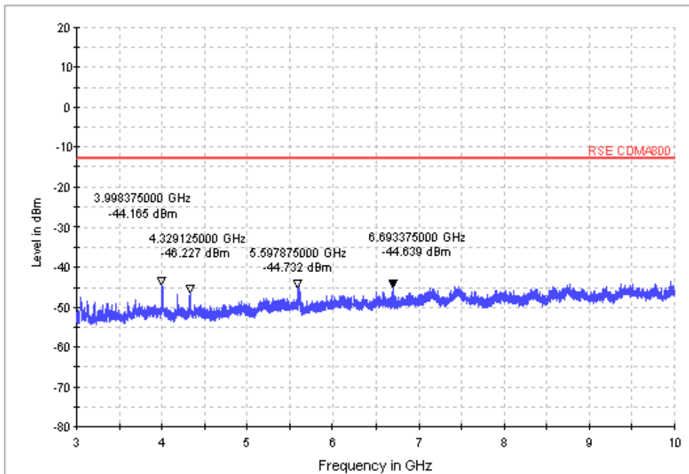
MORLAB-RSE-FCC-CDMA800 3G-10G
