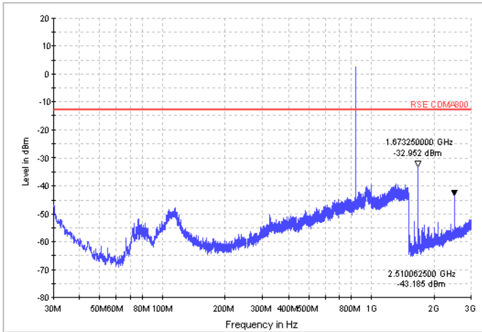
MORLAB-RSE-FCC-CDMA800 30M-3G
