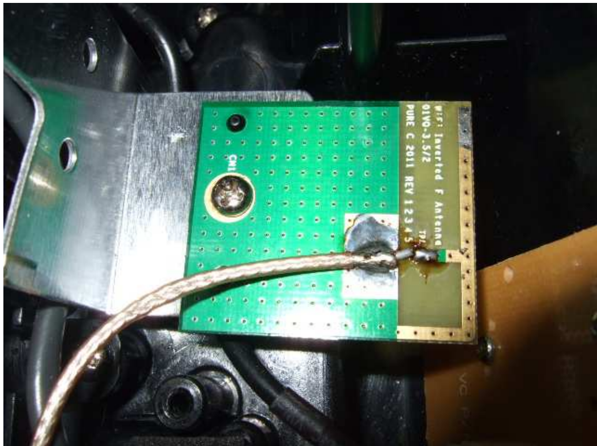
WiFi Antenna:
