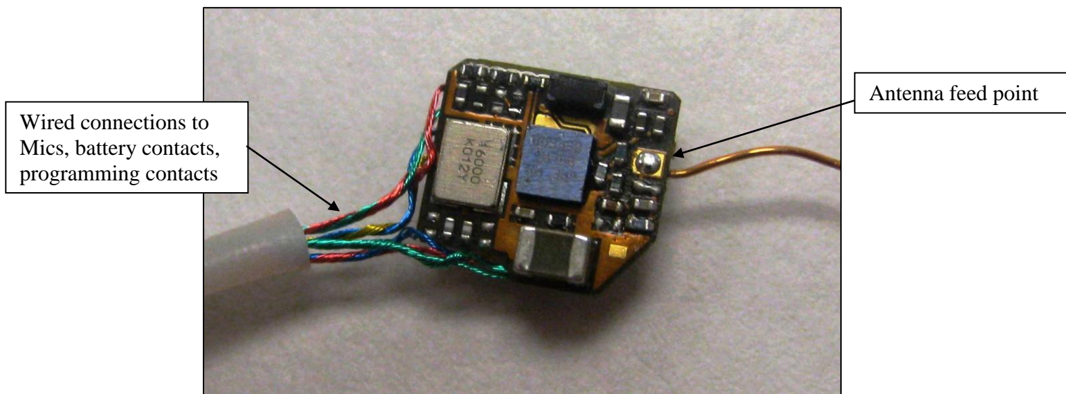
BOTTOM SIDE
