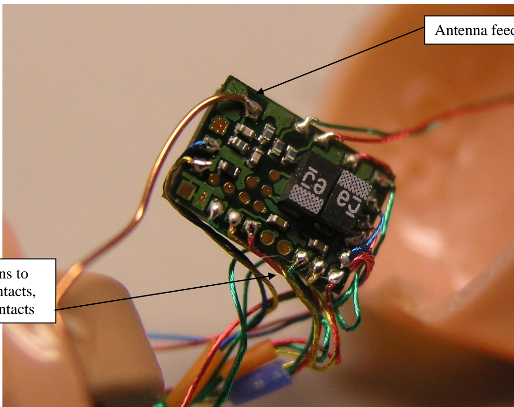
BOTTOM SIDE
