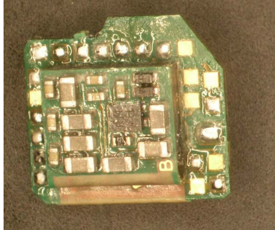
TOP SIDE
