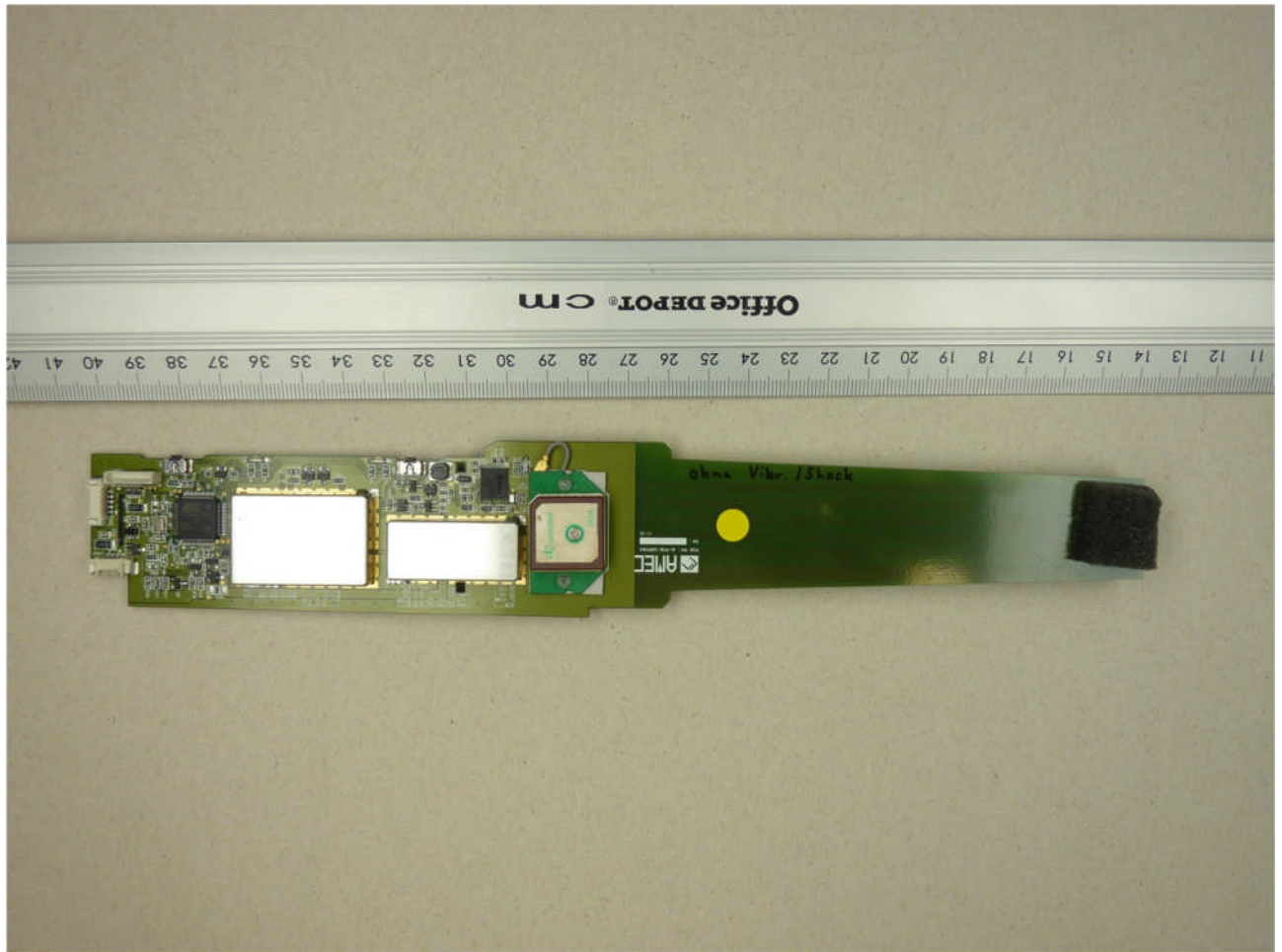
112488eut5.jpg: PCB, front-view
