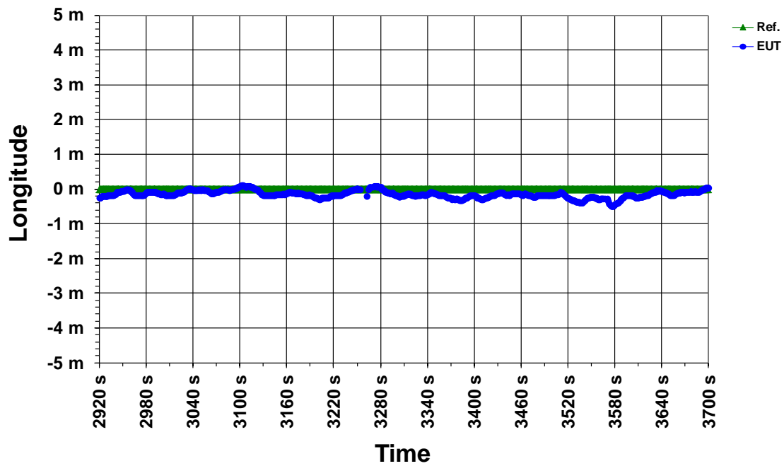
Longitude offset@ 48.6knots vs. time
