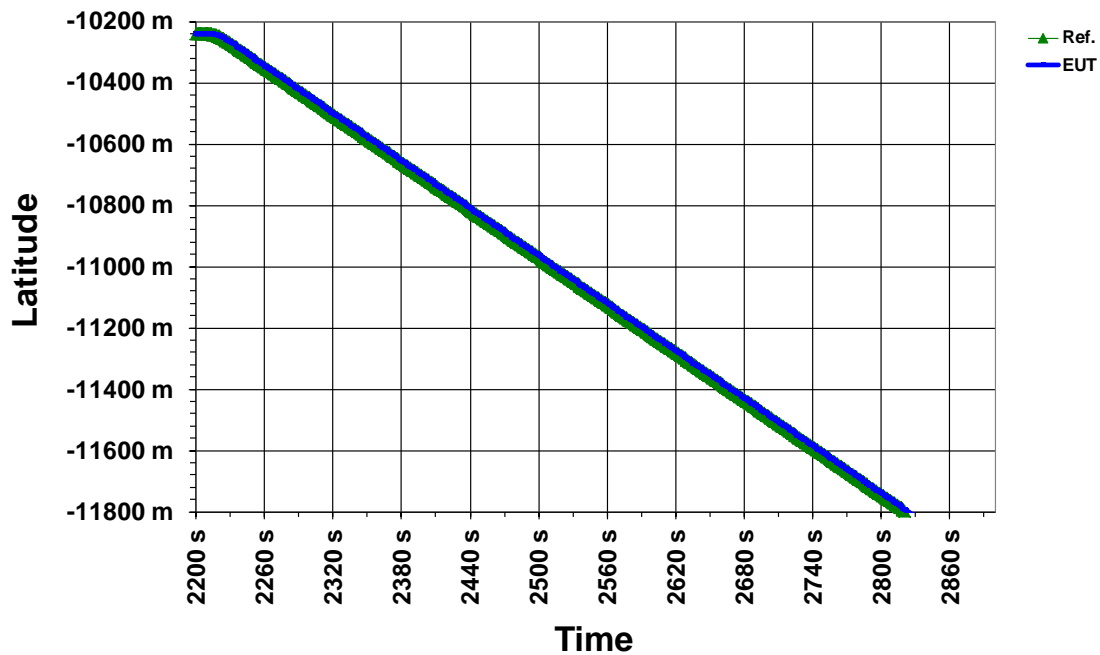
Latitude offset @ 5knots vs. time
