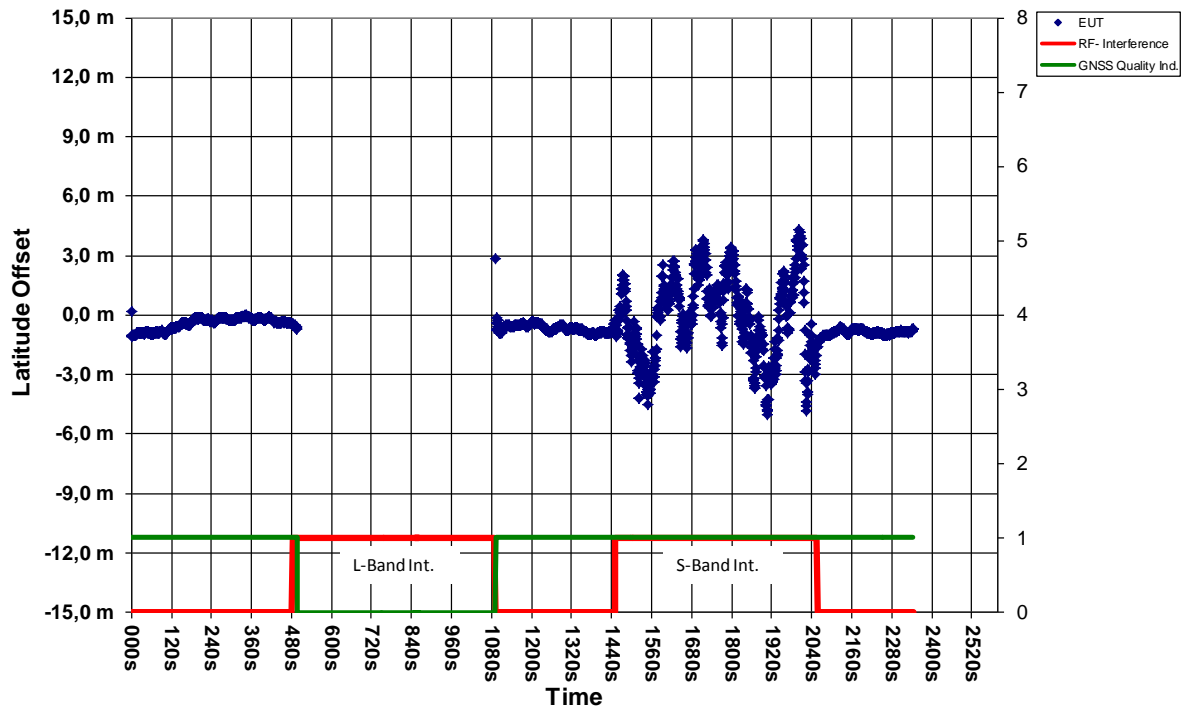
Latitude offset vs. time
