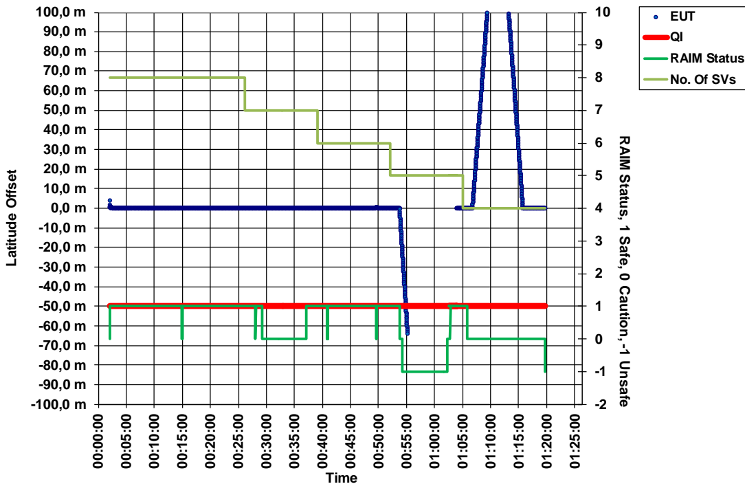
Latitude offset vs. time
