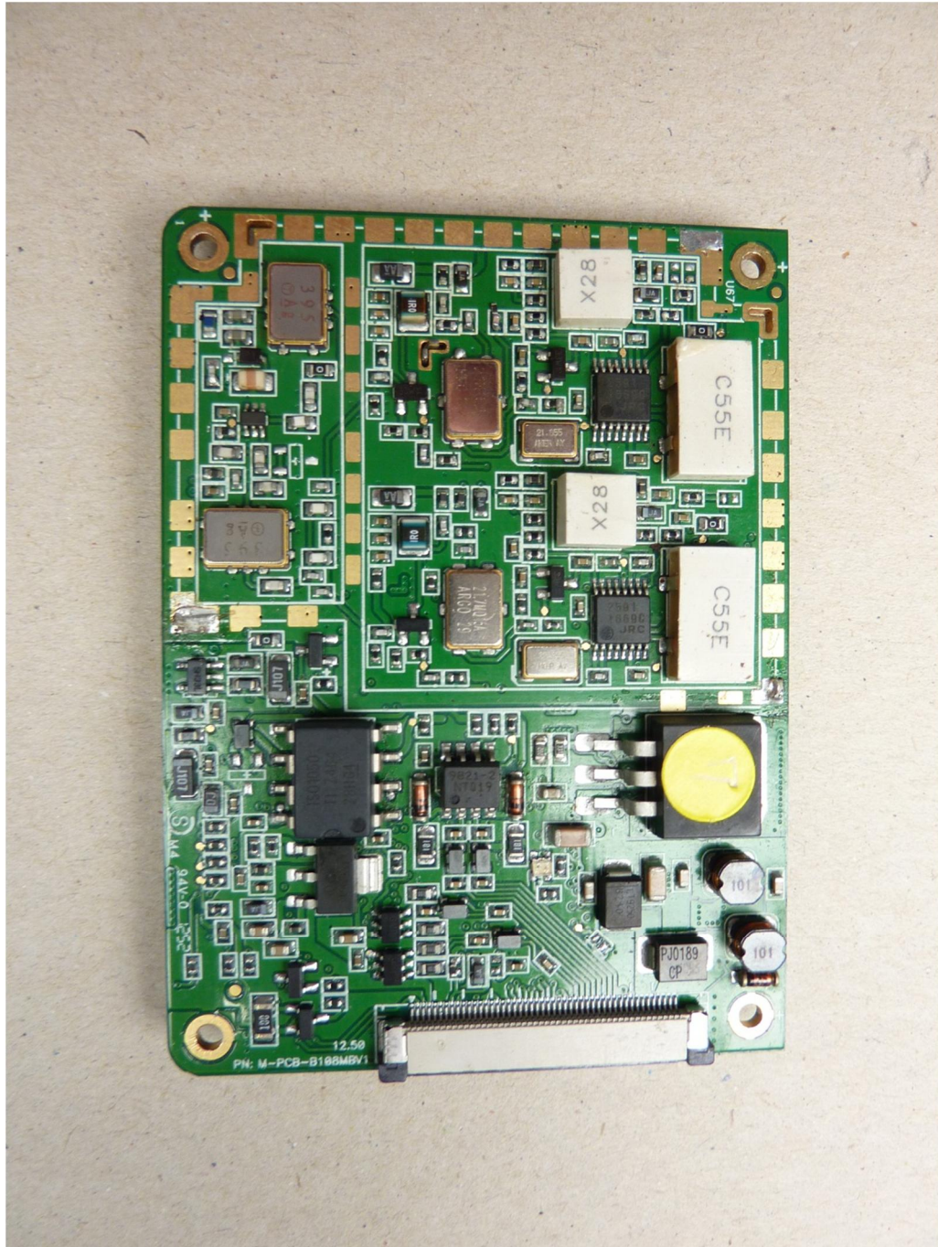
123924eut7.jpg: Main-PCB, front-view
