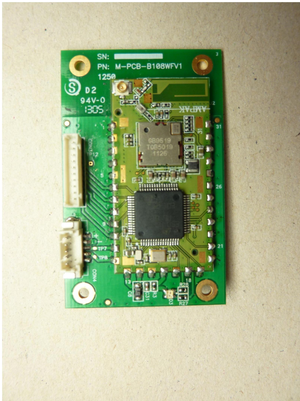
123924eut5.jpg: M-PCB, front-view
