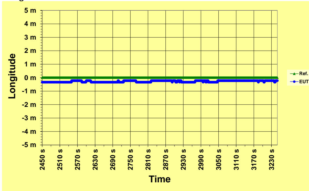
Longitude offset@ 70knots vs. time
