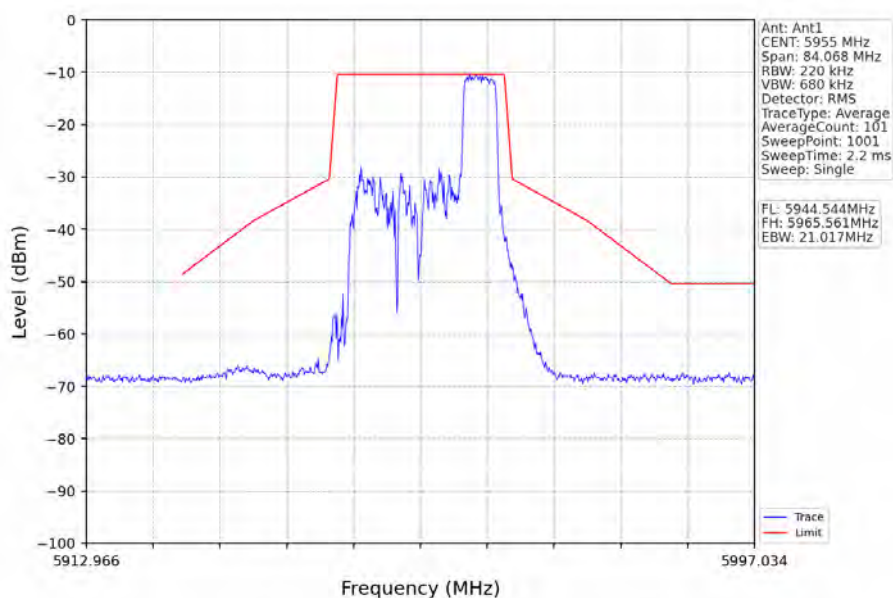
802.11ax(HEW20)_LCH_5955MHz_RU52_Right_Ant1_NTNV
