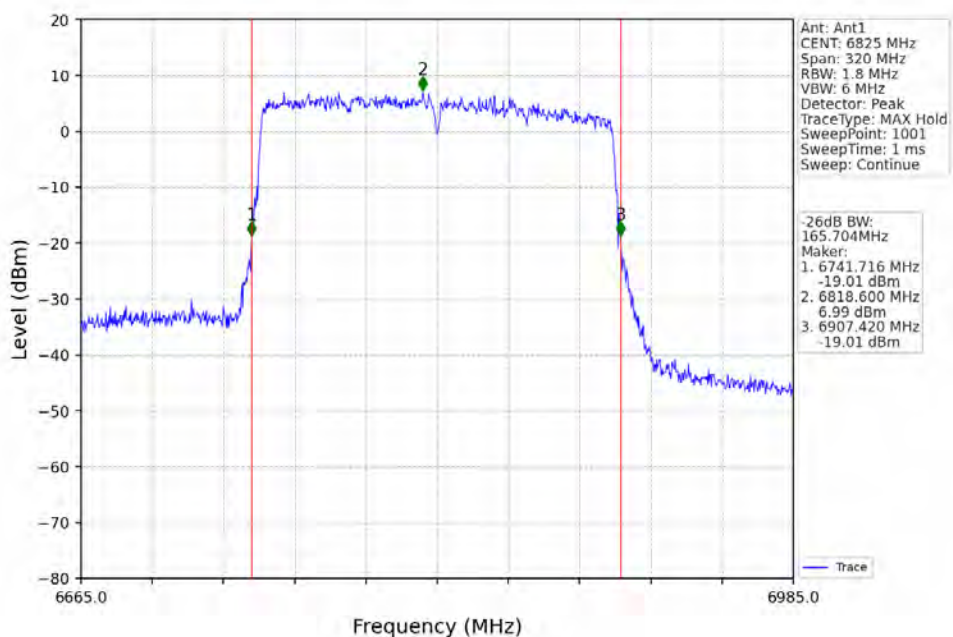
802.11ax(HEW160)_HCH_6825MHz_2xRU996_Left_Ant1_NTNV
