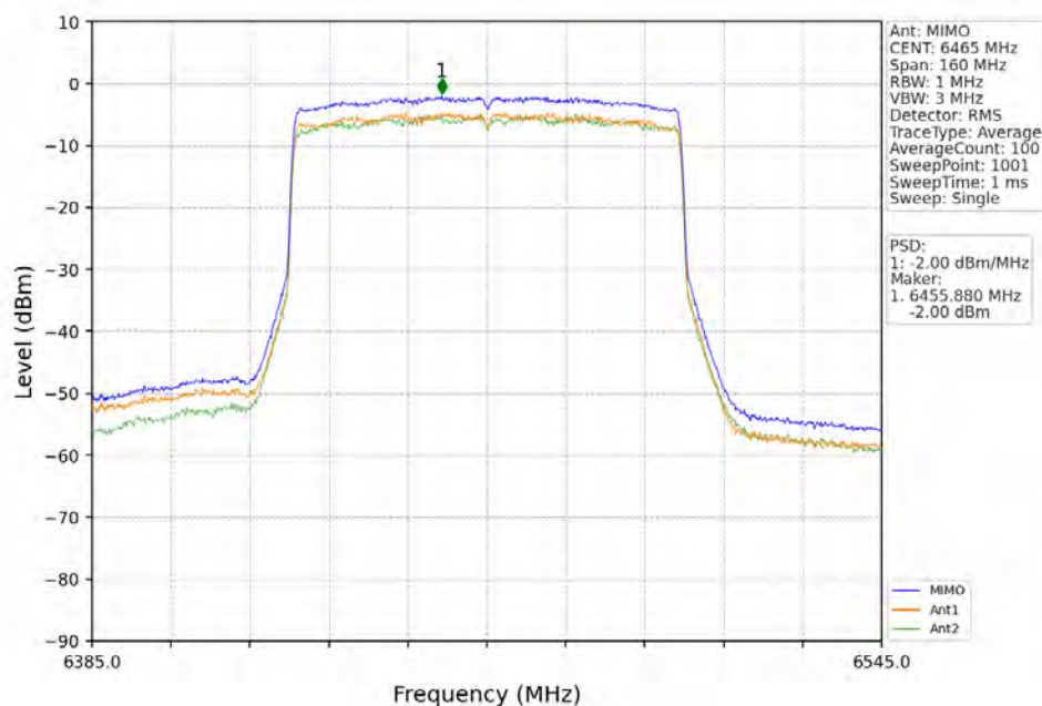
802.11ax(HEW80)_LCH_6465MHz_RU996_Left_MIMO_NTNV
