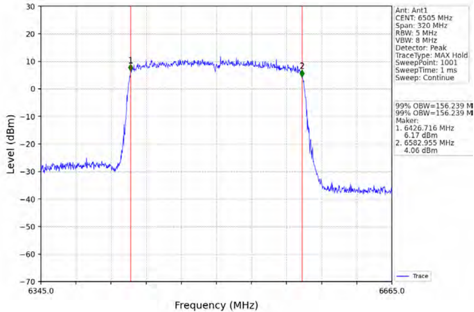
802.11ax(HEW160)_HCH_6505MHz_2xRU996_Left_Ant1_NTNV
