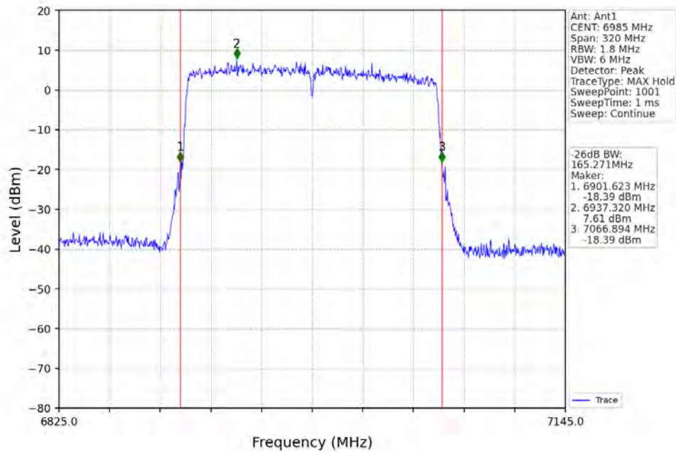
802.11ax(HEW160)_MCH_6985MHz_2xRU996_Left_Ant1_NTNV
