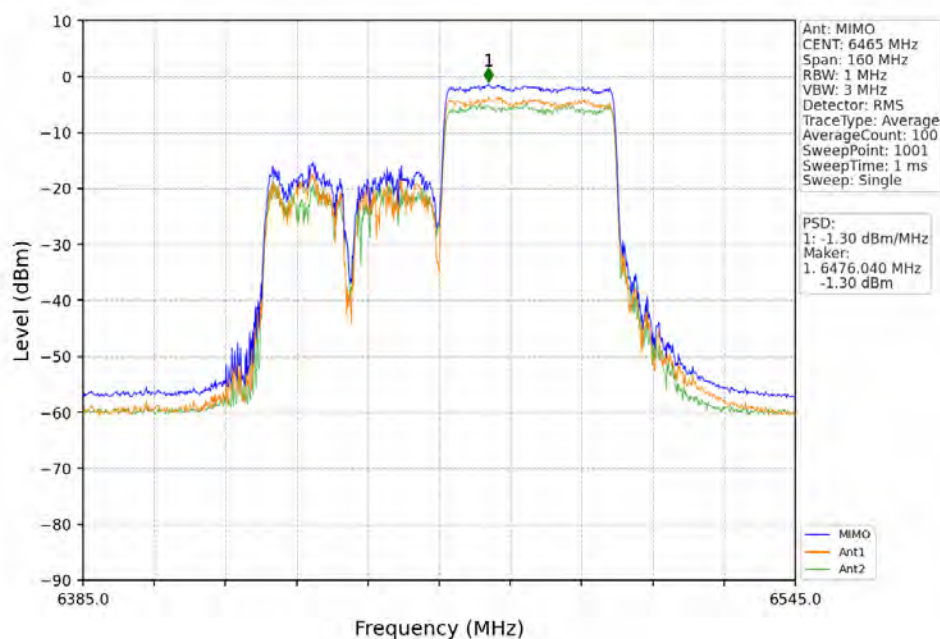
802.11ax(HEW80)_LCH_6465MHz_RU996_Left_MIMO_NTNV
