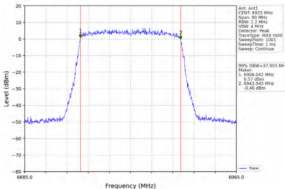
802.11ax(HEW40)_LCH_6925MHz_RU484_Left_Ant1_NTNV
