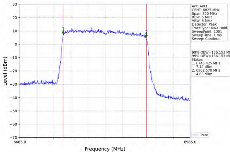
802.11ax(HEW160)_HCH_6825MHz_2xRU996_Left_Ant1_NTNV
