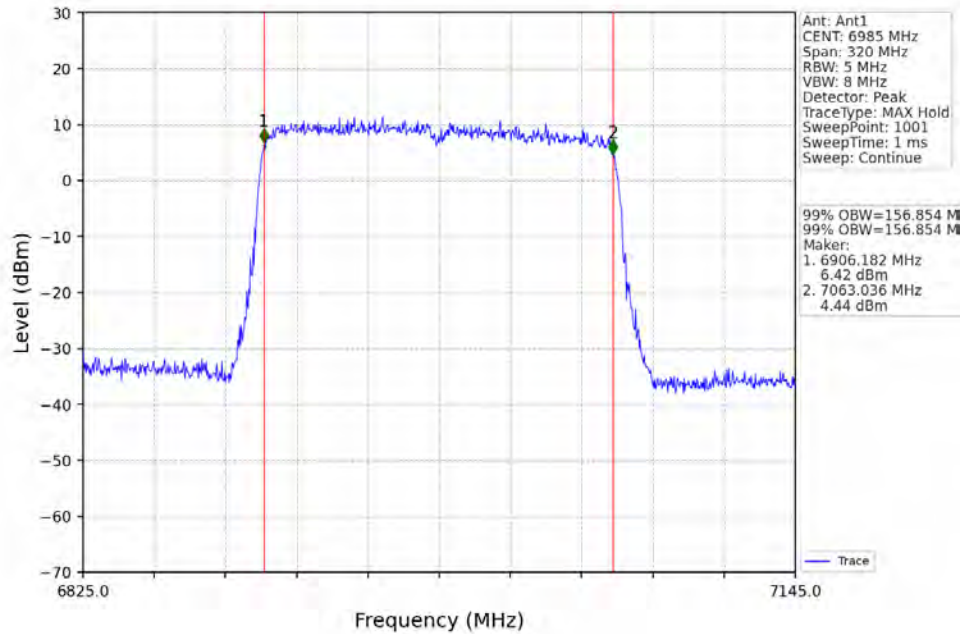
802.11ax(HEW160)_MCH_6985MHz_2xRU996_Left_Ant1_NTNV
