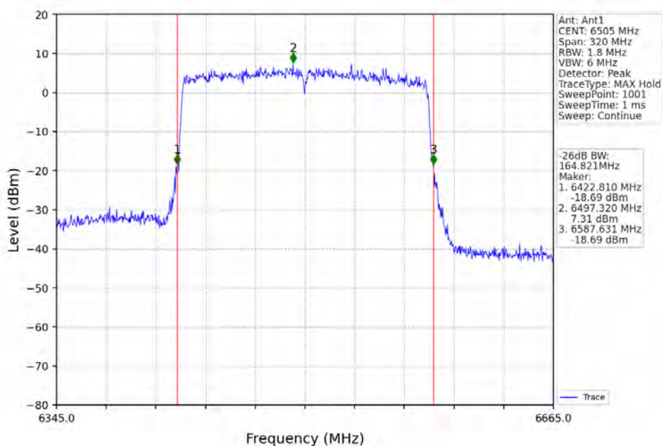
802.11ax(HEW160)_HCH_6505MHz_2xRU996_Left_Ant1_NTNV
