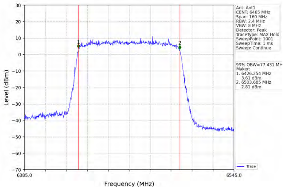
802.11ax(HEW80)_LCH_6465MHz_RU996_Left_Ant1_NTNV
