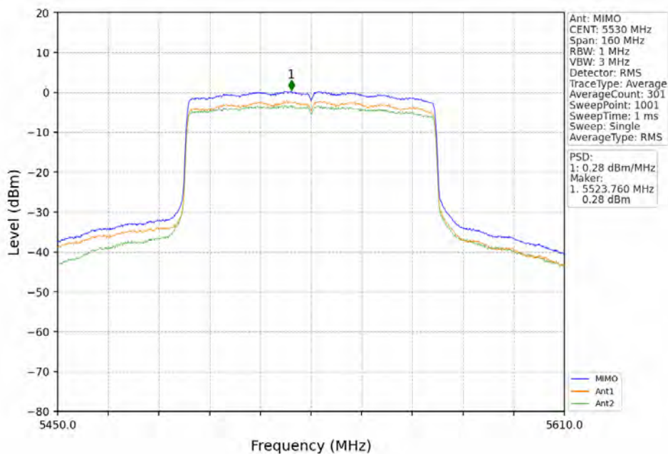
802.11ax(HEW80)_LCH_5530MHz_RU996_Left_MIMO_NTNV
