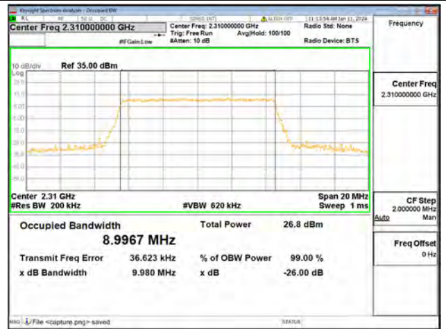
B30 / 10MHz / 256QAM / Mid CH
