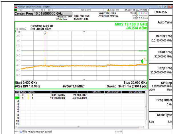
n77(3700-3980MHz) (30MHz-20GHz) 20M DFT-s-OFDM BPSK Edge 1RB Left Mid
