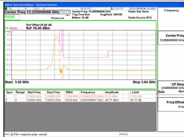
B42(3550-3600) / 20MHz / High CH / QPSK / 1 RB
