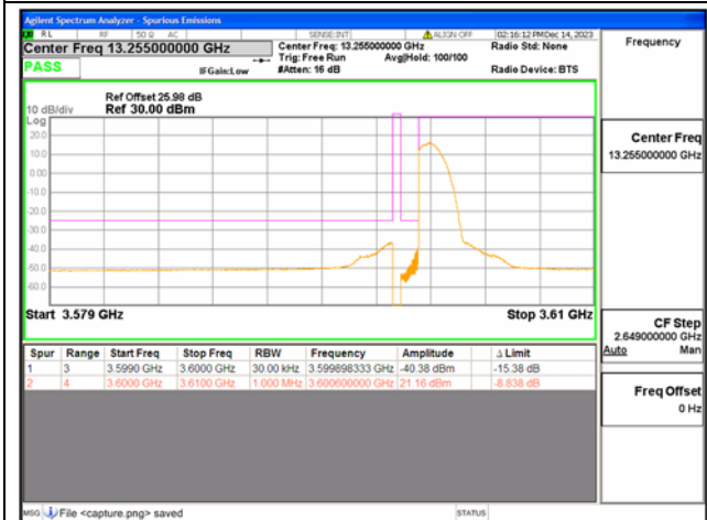
B43(3600-3700) / 10MHz / Low CH / QPSK / 1 RB
