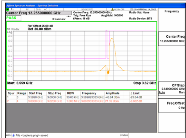
B43(3600-3700) / 20MHz / Low CH / QPSK / 1 RB
