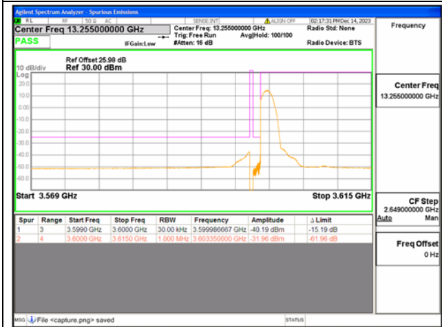
B43(3600-3700) / 15MHz / Low CH / QPSK / 1 RB
