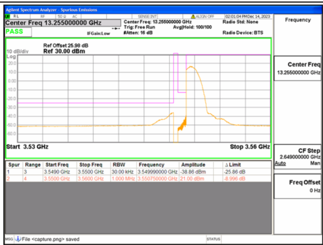
B42(3550-3600) / 5MHz / Low CH / QPSK / 1 RB
