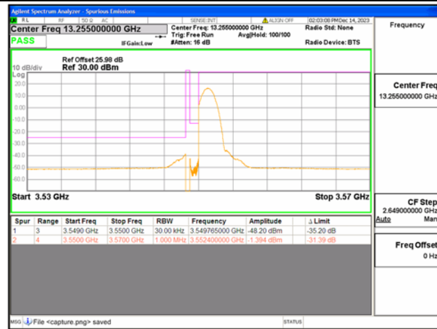
B42(3550-3600) / 20MHz / Low CH / QPSK / 1 RB
