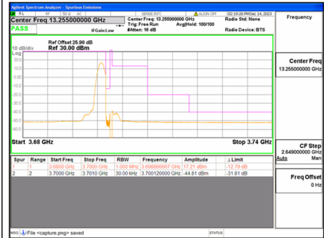
B43(3600-3700) / 20MHz / High CH / QPSK / 1 RB
