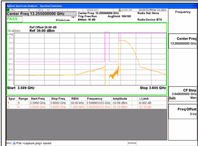
B43(3600-3700) / 5MHz / Low CH / QPSK / 1 RB
