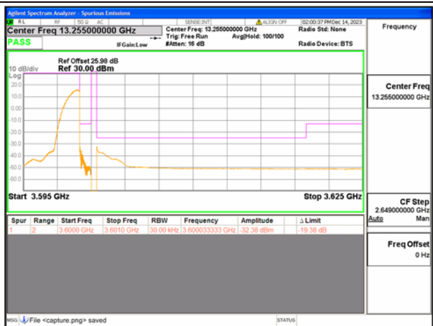
B42(3550-3600) / 5MHz / High CH / QPSK / 1 RB
