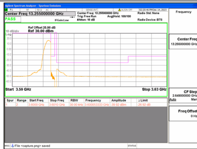
B42(3550-3600) / 10MHz / High CH / QPSK / 1 RB
