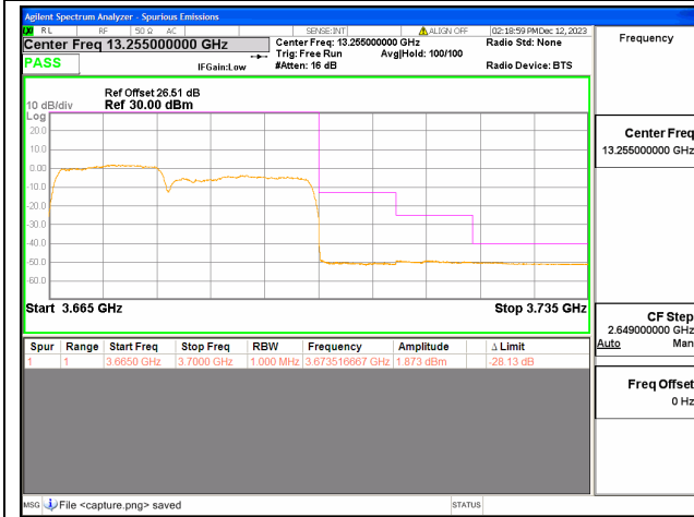
48C / 15+20MHz / High CH / QPSK / 75#0-100#0
