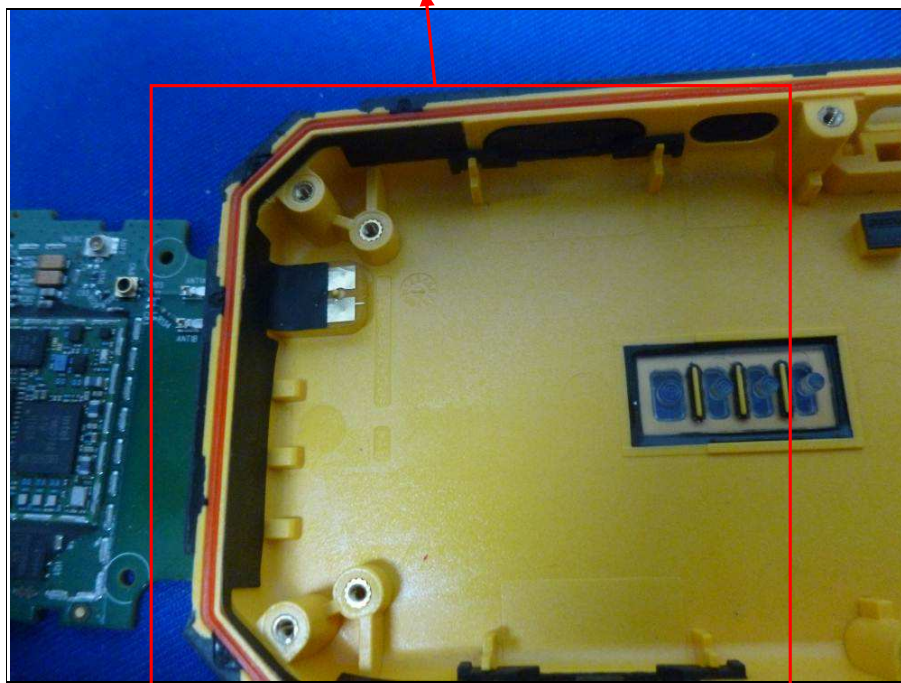
WWAN Antenna
