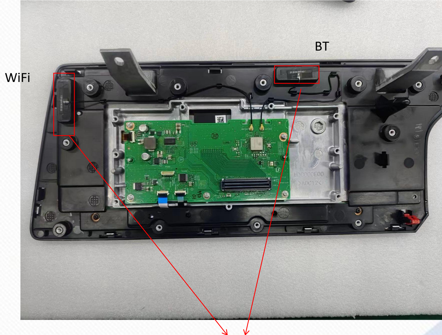
天线贴装位置
