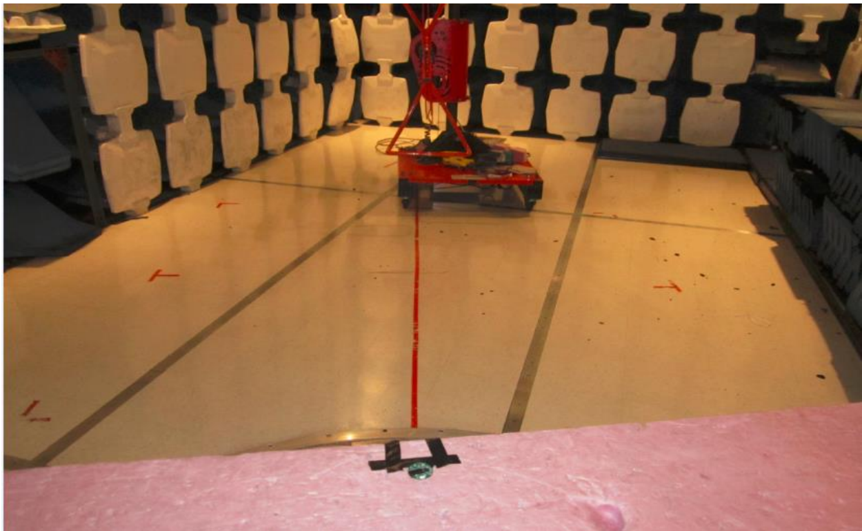
30-1000MHz
