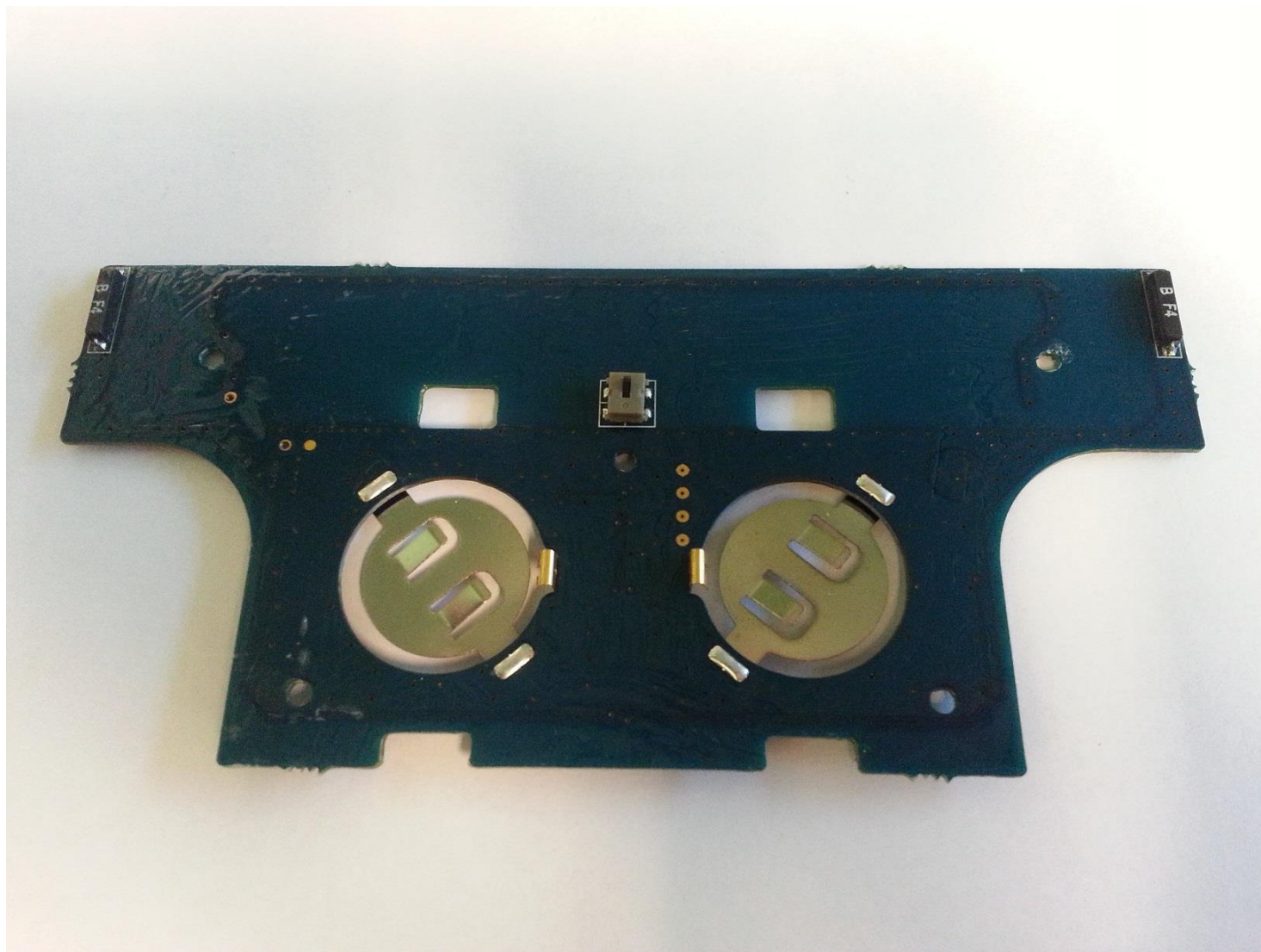
Hinge Door PCB – BACK
