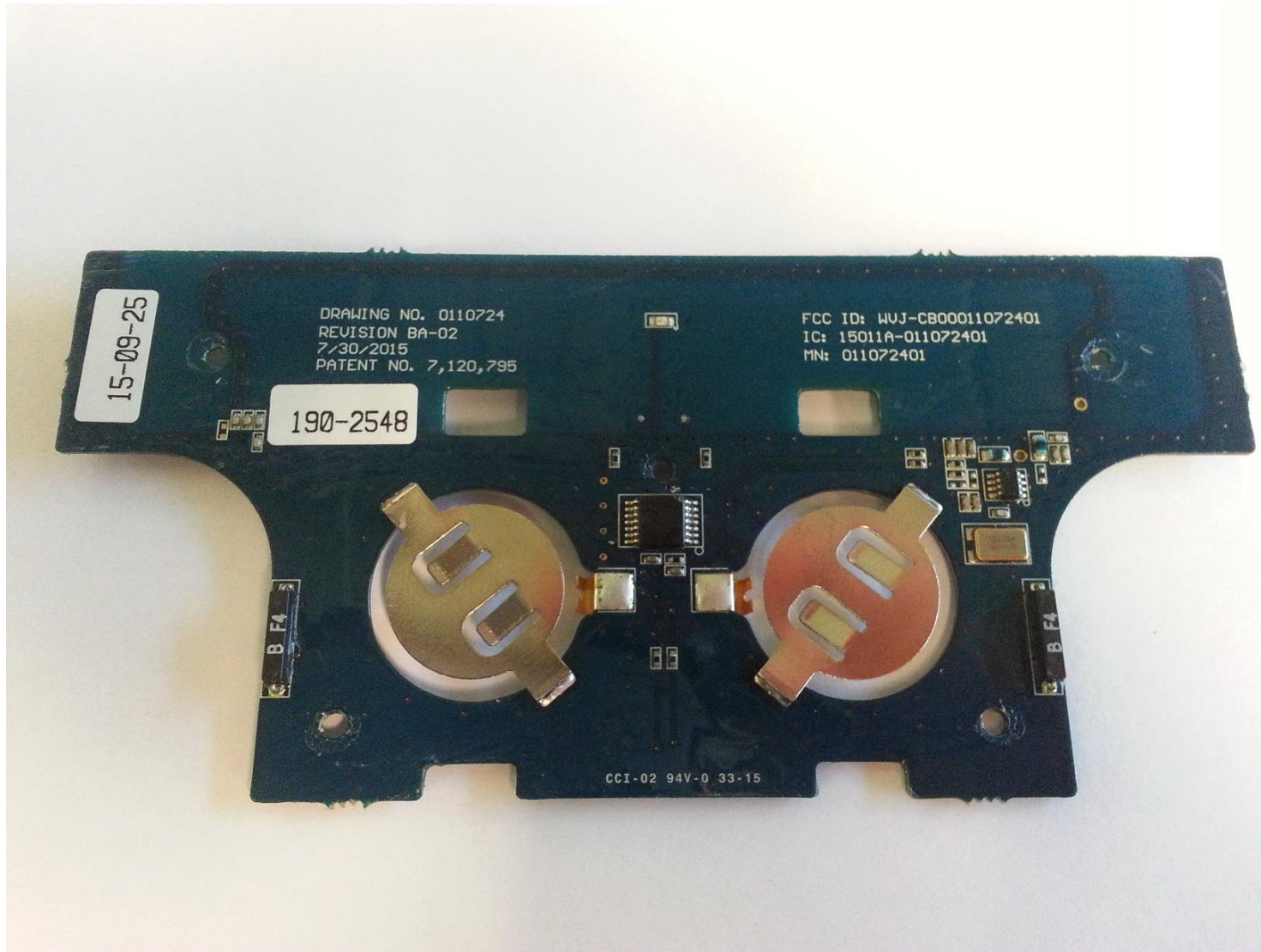
Hinge Door PCB – FRONT
