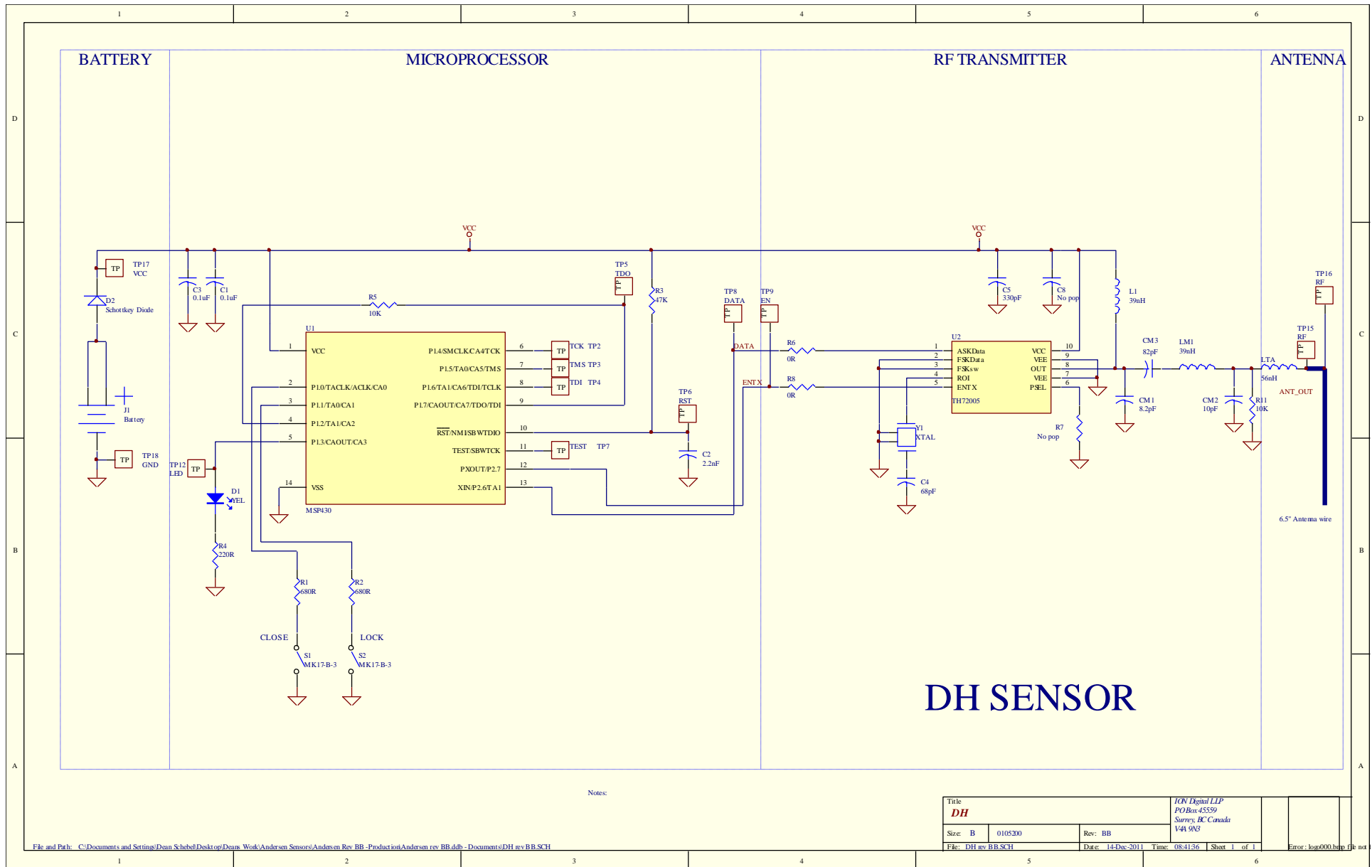
DH Rev BB Schematic – Dec 14 2011
