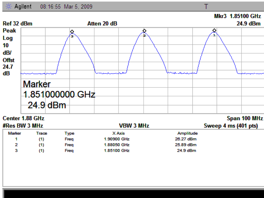
(Plot A: CDMA 1900MHz Channel = 25, 600, 1175)
