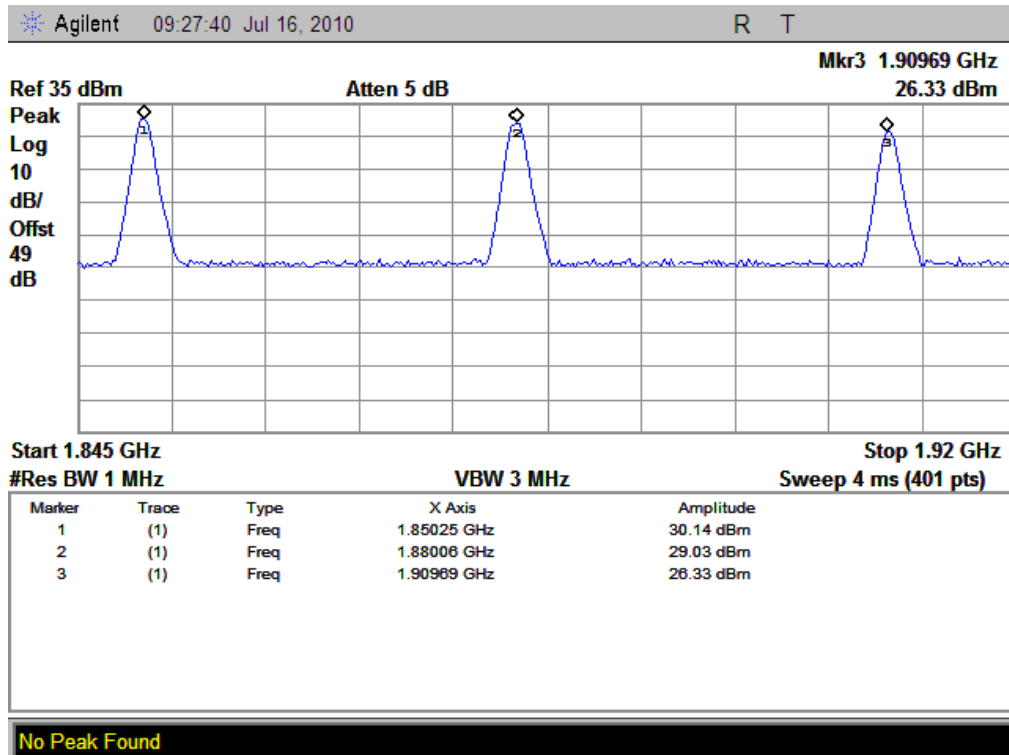
(Plot D: GPRS-2TX 1900MHz Channel = 512, 661, 810)
