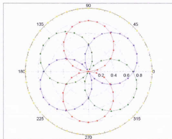
f=1800 MHz,R22
