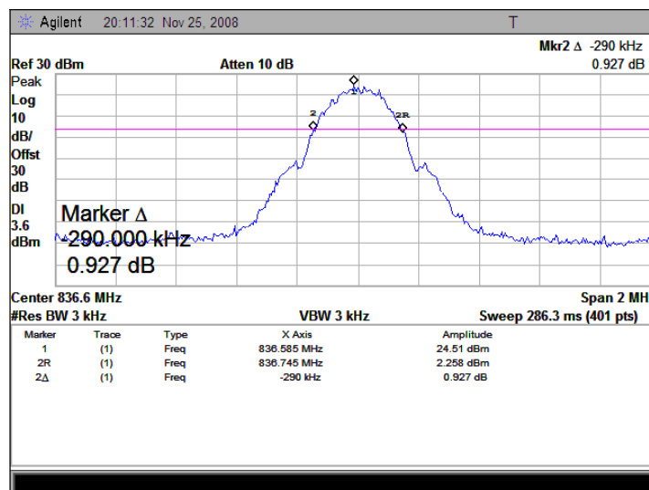
(Plot B: GSM 850MHz Channel = 190)
