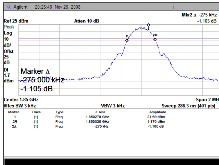
(Plot D: GSM 1900MHz Channel = 512)
