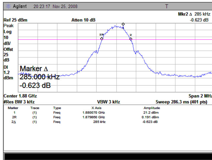
(Plot E: GSM 1900MHz Channel = 661)
