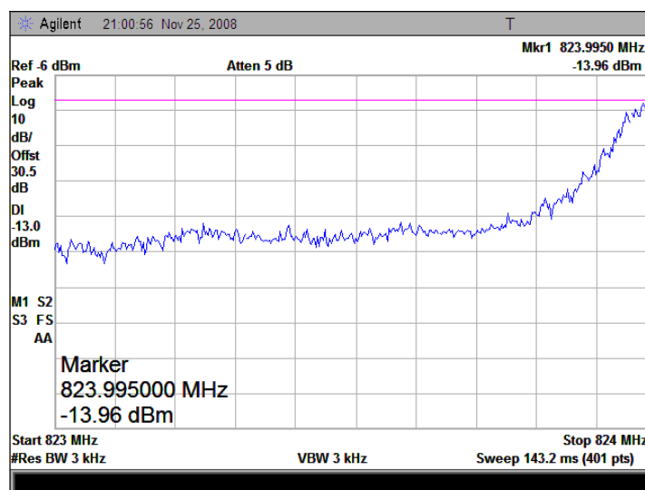
(Plot A: Channel = 128)
