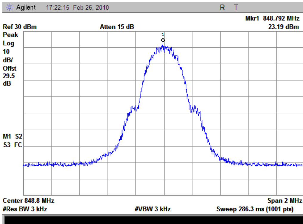
(Plot B: GSM 850MHz Channel = 251)
