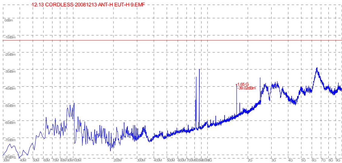
(Plot A: Test Antenna Horizontal)
