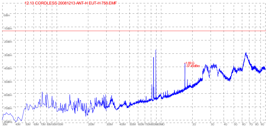
(Plot A: Test Antenna Horizontal)
