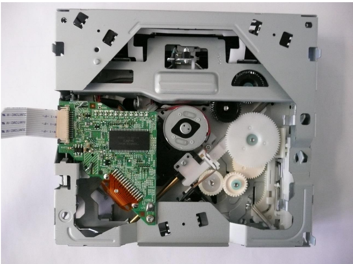
CD-PCB 01
