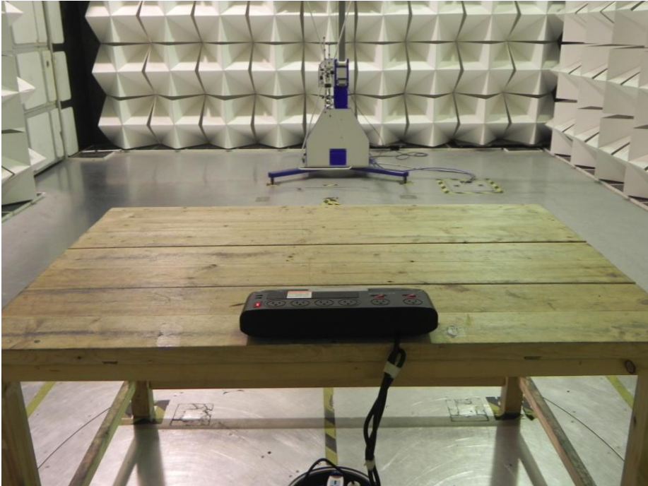
30MHz~1000MHz
