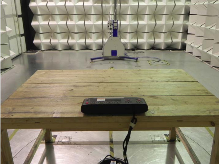
30MHz~1000MHz
