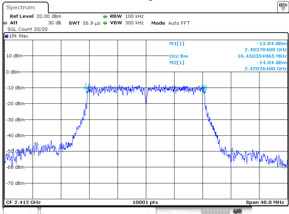
6dB NVNT 802.11g 2412MHz Ant1
