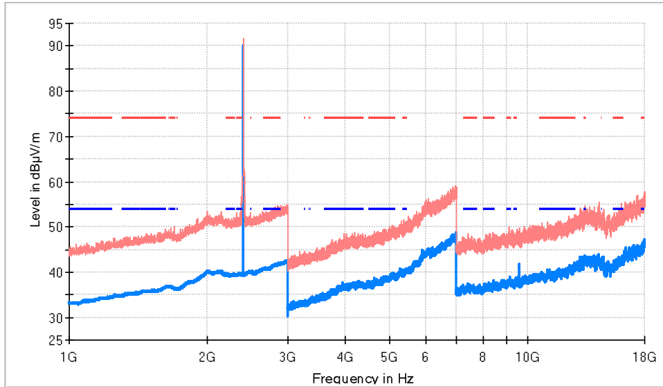
1GHz_18GHz_HP & VP_CH Low
