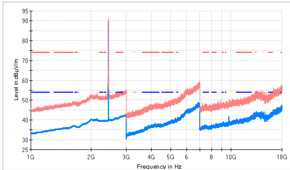
1GHz_18GHz_HP & VP_CH Mid
