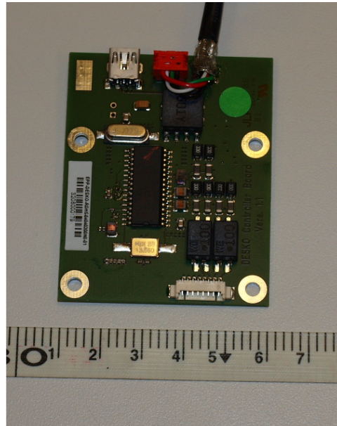
Picture 1-1: RFID 500 module top side
