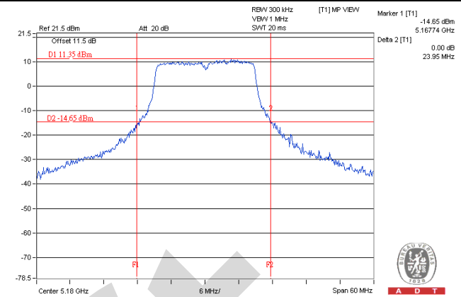
802.11ac (20MHz)
