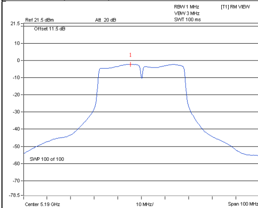
802.11ac (40MHz)
