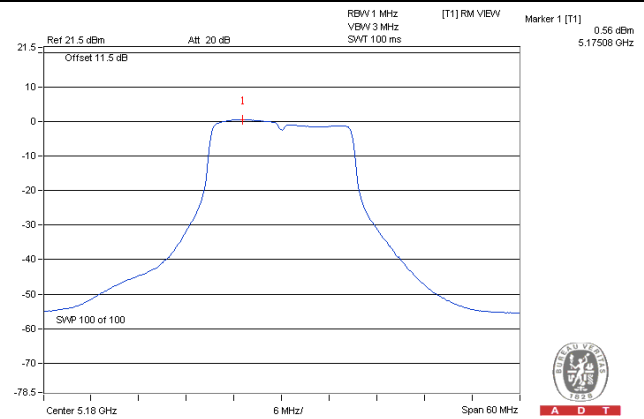
802.11ac (20MHz)
