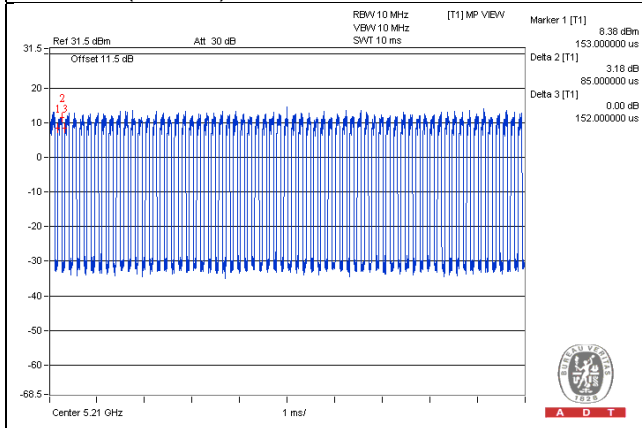
802.11ac (80MHz)
