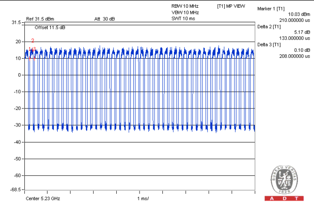
802.11ac (40MHz)
