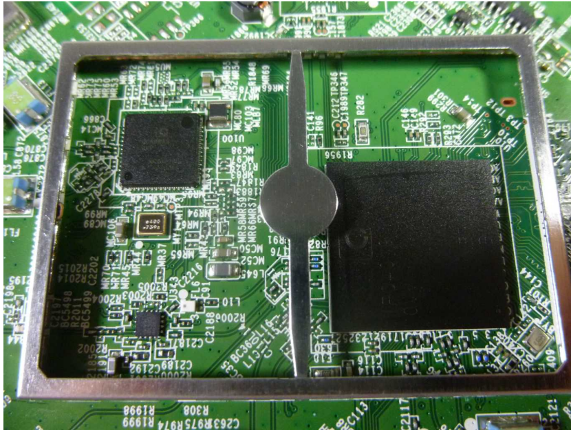
Photo 5 EUT ICs
