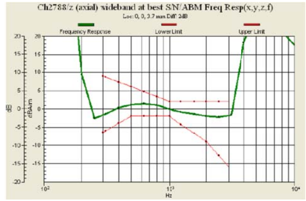
Fig. 7.6 WCDMA Band VIII Ch2788
