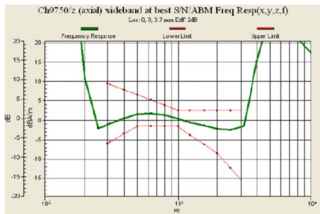
Fig. 7.8 WCDMA Band I Ch9750
