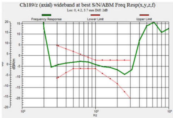
Fig 7.1 GSM850 Ch189
