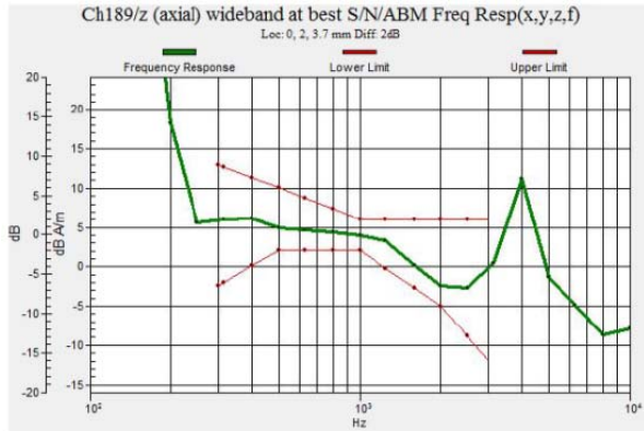
Fig. 9.1 GSM850 Ch189
