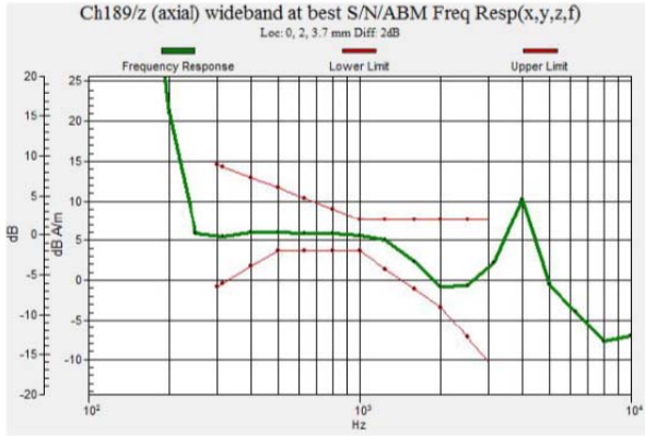
Fig. 9.5 GSM850 Ch189
