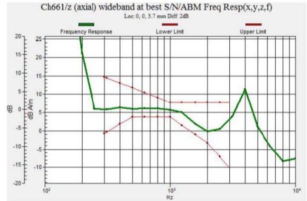
Fig. 9.6 GSM1900 Ch661
