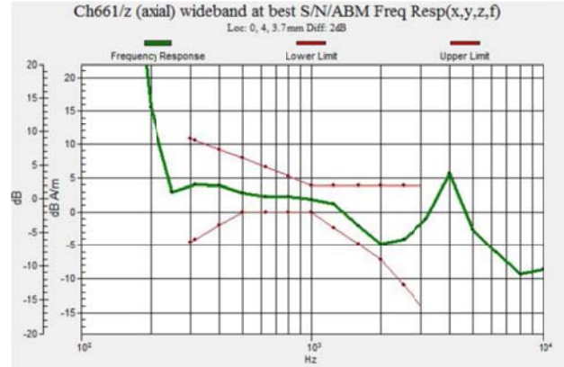
Fig. 9.6 GSM1900 Ch661
