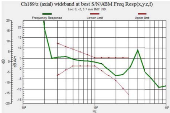
Fig. 9.10 GSM850 Ch189
