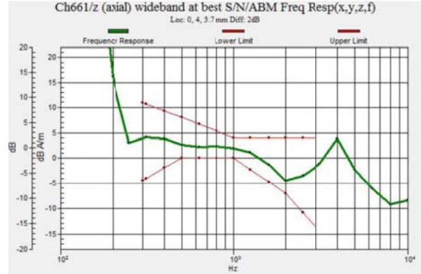
Fig. 9.2 GSM1900 Ch661
