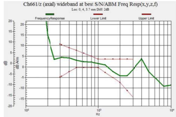
Fig. 9.11 GSM1900 Ch661
