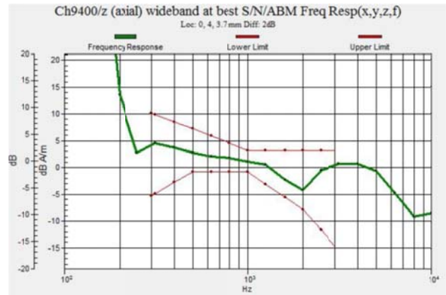
Fig. 9.4 WCDMA Band II Ch9400
