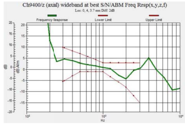
Fig. 9.13 WCDMA Band II Ch9400
