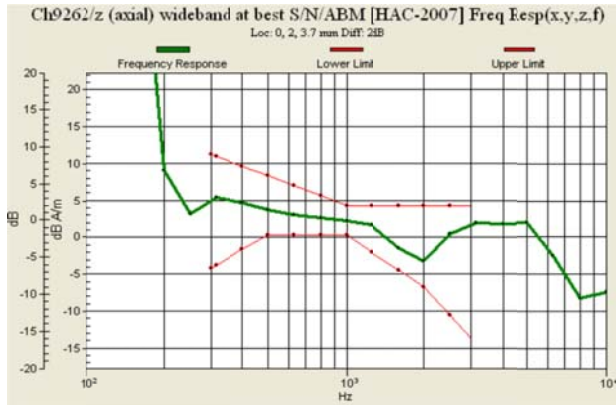
Fig. 9.7 WCDMA Band II Ch9262
