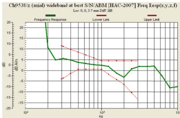
Fig. 9.9 WCDMA Band II Ch9538
