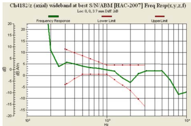
Fig. 9.11 WCDMA Band V Ch4182
