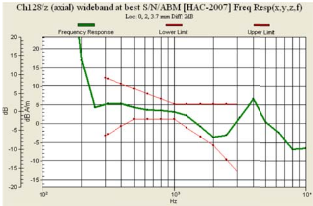
Fig. 9.1 GSM850 Ch128
