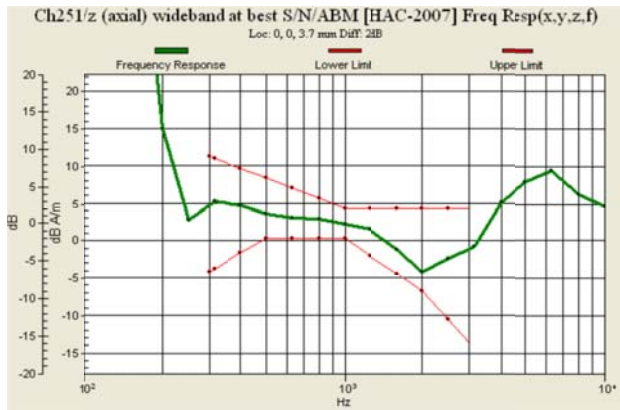
Fig. 9.3 GSM850 Ch251
