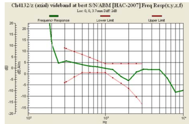
Fig. 9.10 WCDMA Band V Ch4132
