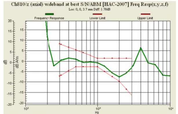
Fig. 9.6 GSM1900 Ch810
