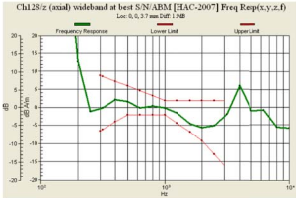
Fig. 9.1 GSM850 Ch128
