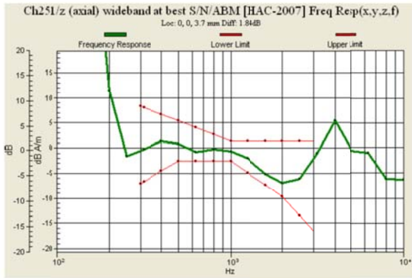
Fig. 9.3 GSM850 Ch251
