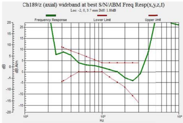
Fig. 9.1 GSM850 Ch189
