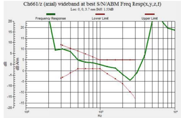
Fig. 9.2 GSM1900 Ch661
